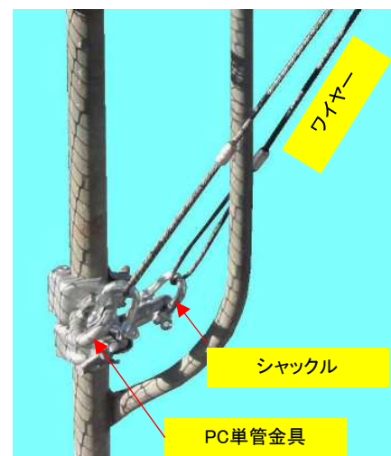
4 PC単管金具 + シャックル + ワイヤー
