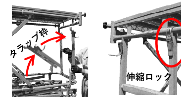
タラップ枠を起し、伸縮ロックを掛ける
