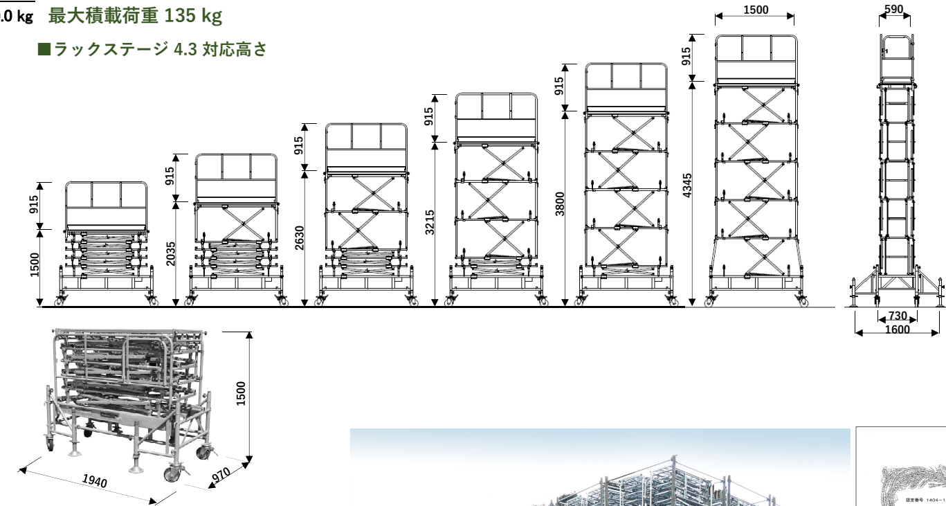
収納ロックを外し伸ばす
